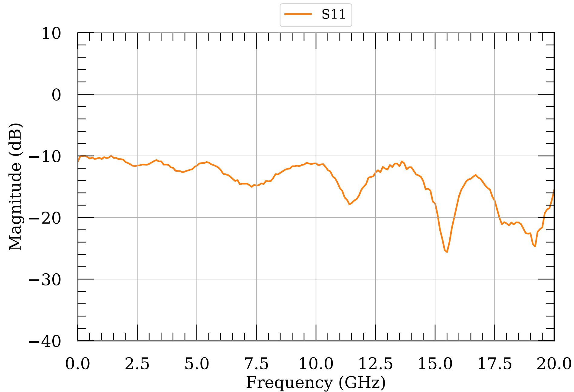
LNA S-params module017
